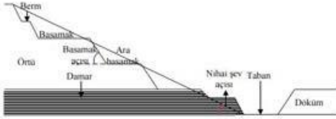
Şekil 2.9. Açık işletme kesit görünümü [4]
