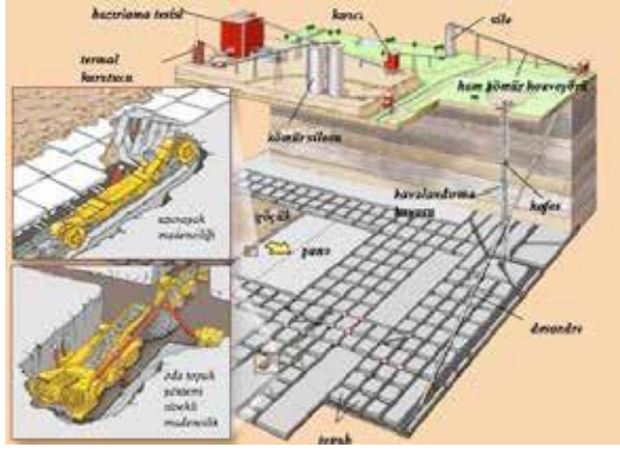
Şekil 2.3. Uzunayak madenciliği ve oda topuk yöntemi görseli
